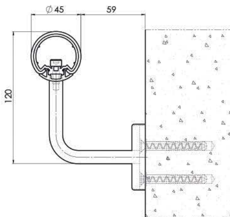
nerezová rúčka stainless steel handle
